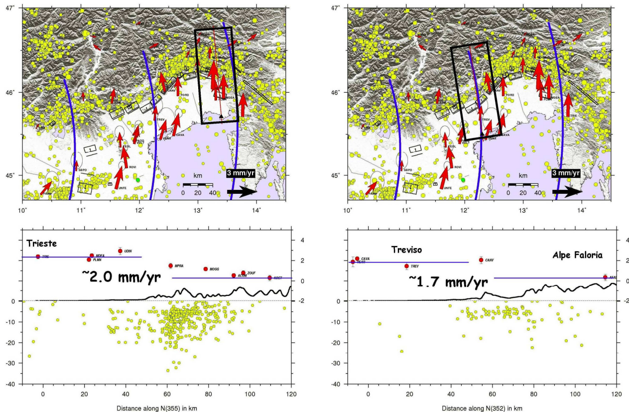
Fig. 5 - Accumulo di deformazione attraverso le Alpi Meridionali, con evidenziate l'area Trieste- Salzburg e Treviso-Belluno (E. Serpelloni –2008)
