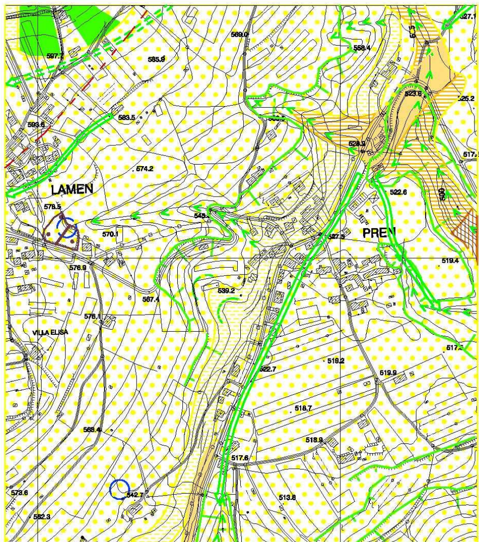
Tavola n.2 : Elementi geologici in chiave sismologica
