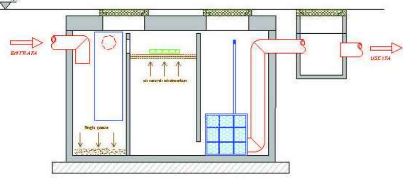
Schema impianto desolatore e desabbiatore
